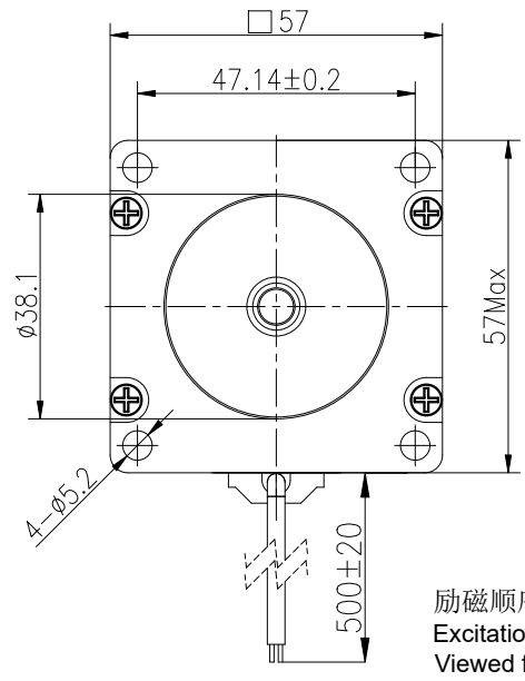
电机接线 Motor Wiring Diagram
